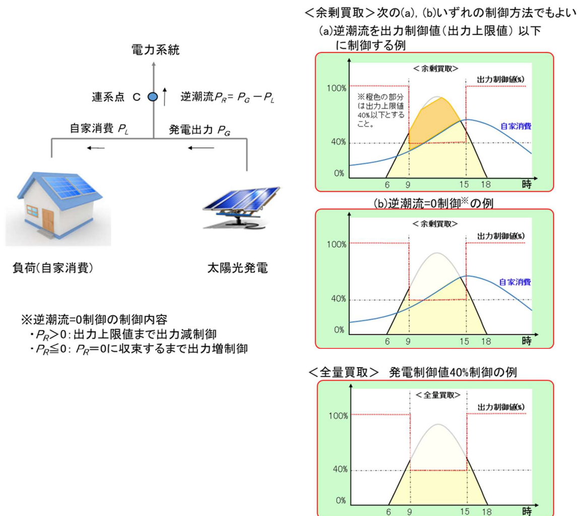
図 4.4 余剰買取制御（太陽光発電の例）
