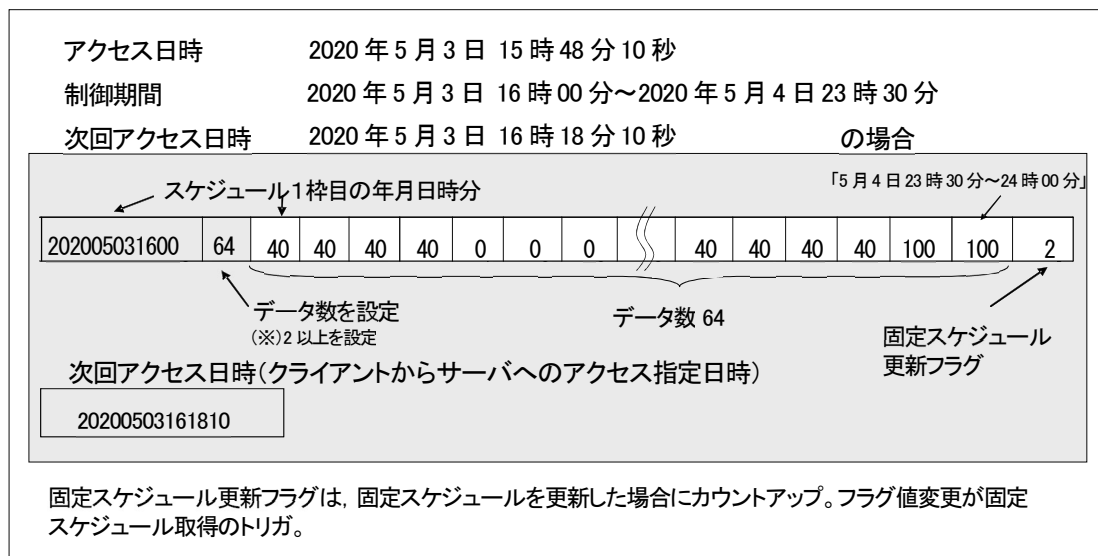
図 8.4 更新スケジュールのデータ構造
