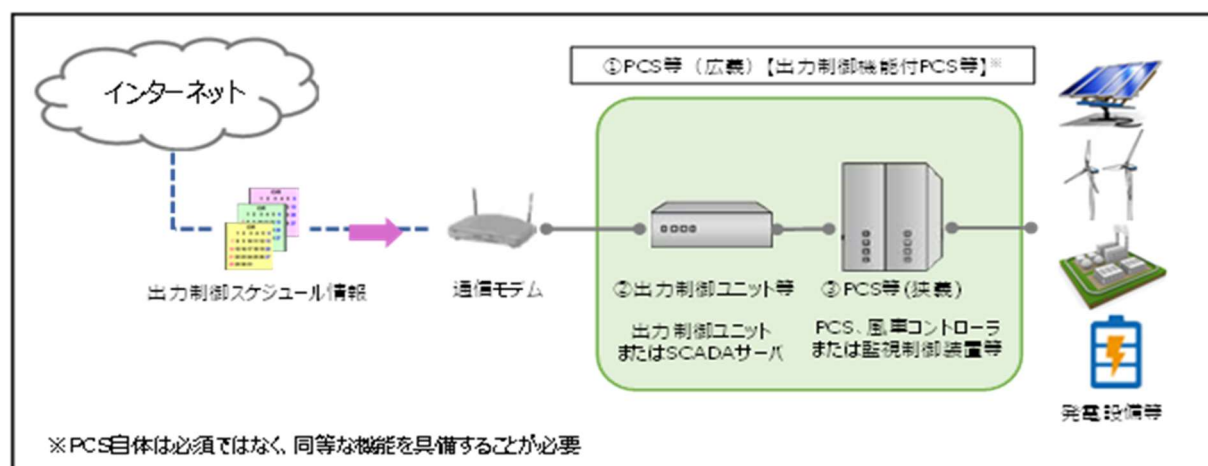
図 3.1 出力制御機能付 PCS 等 システムの構成
