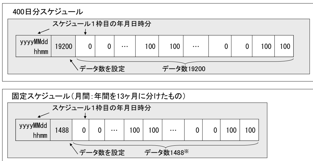
図 8.2 固定スケジュールのデータ構造
