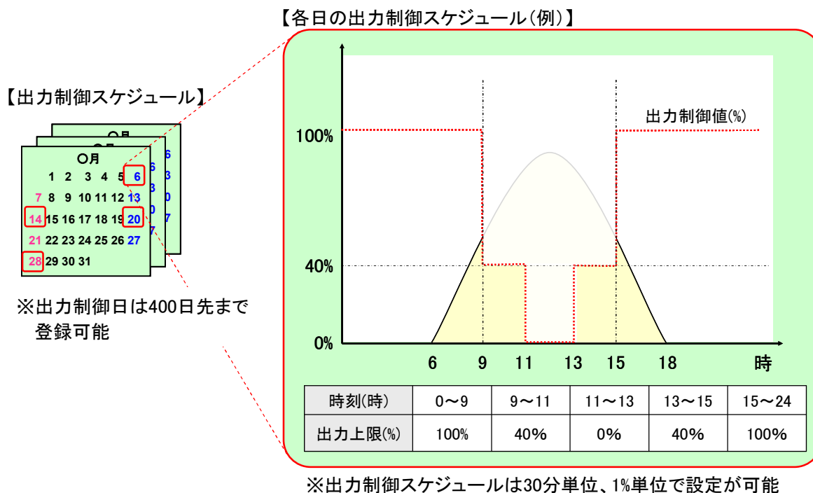
図 4.2 スケジュール設定内容
