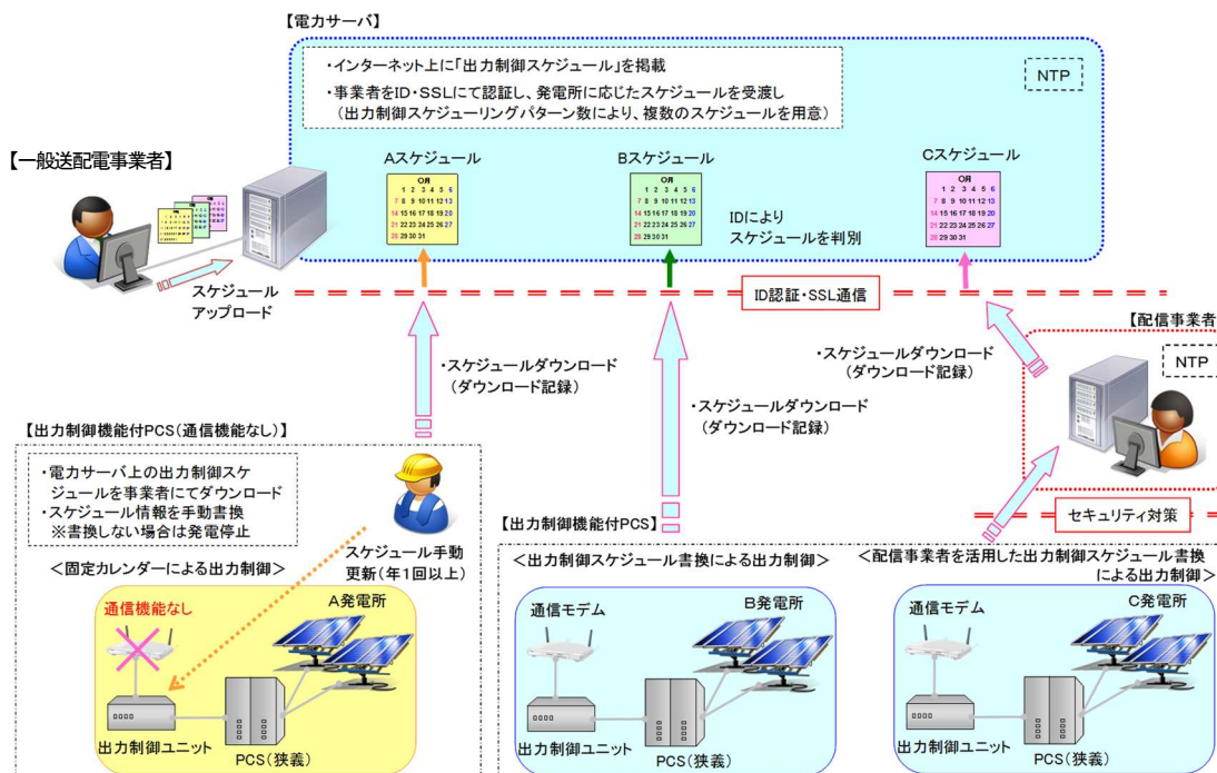
図 4.1 出力制御スケジュールの書換の仕組み（太陽光発電の例）
