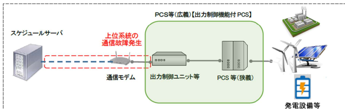
・ 図 7.3 上位系統の通信故障
