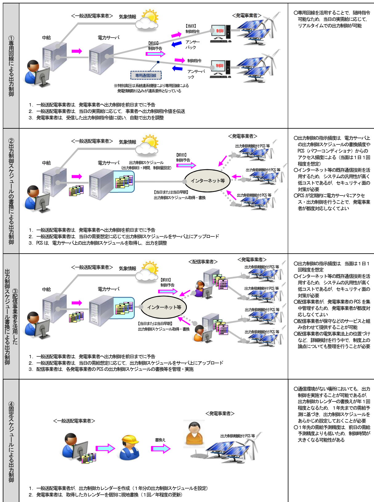
図 2.1 出力制御システムの概要
