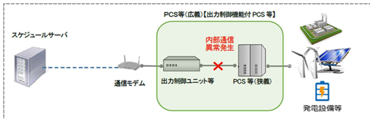
図 6.1 内部通信異常
